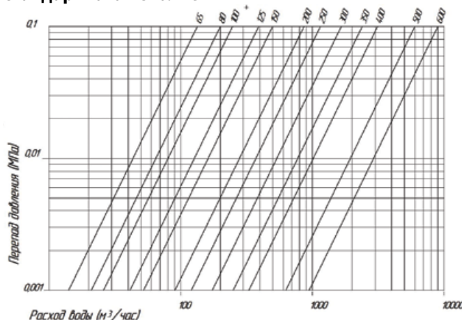
Диаграмма перепада давления для фильтра стандартного исполнения
