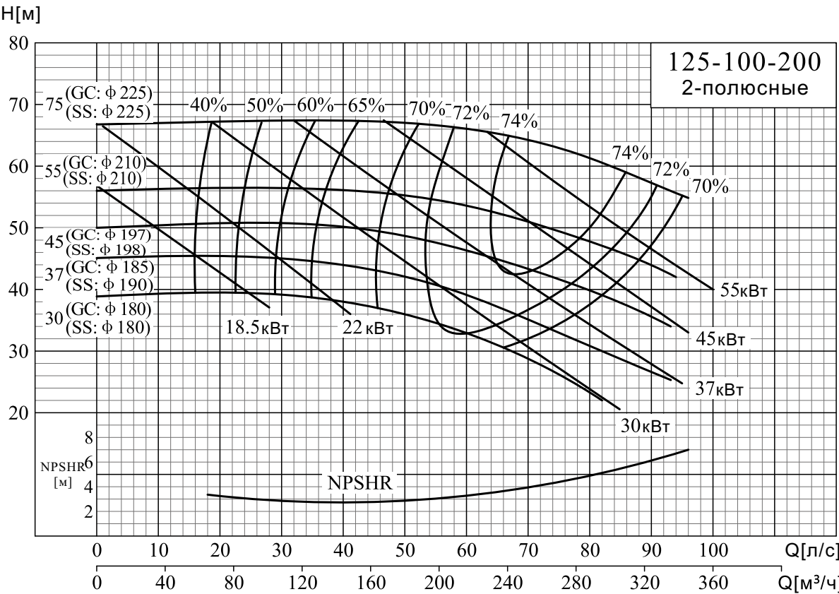
NISO,NIS,NISF125-100-200/125-100-250
