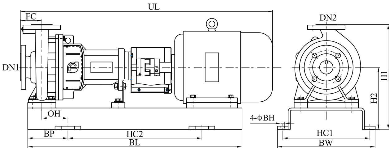
Габаритно-присоединительные размеры насосного агрегата в сборе NISO
