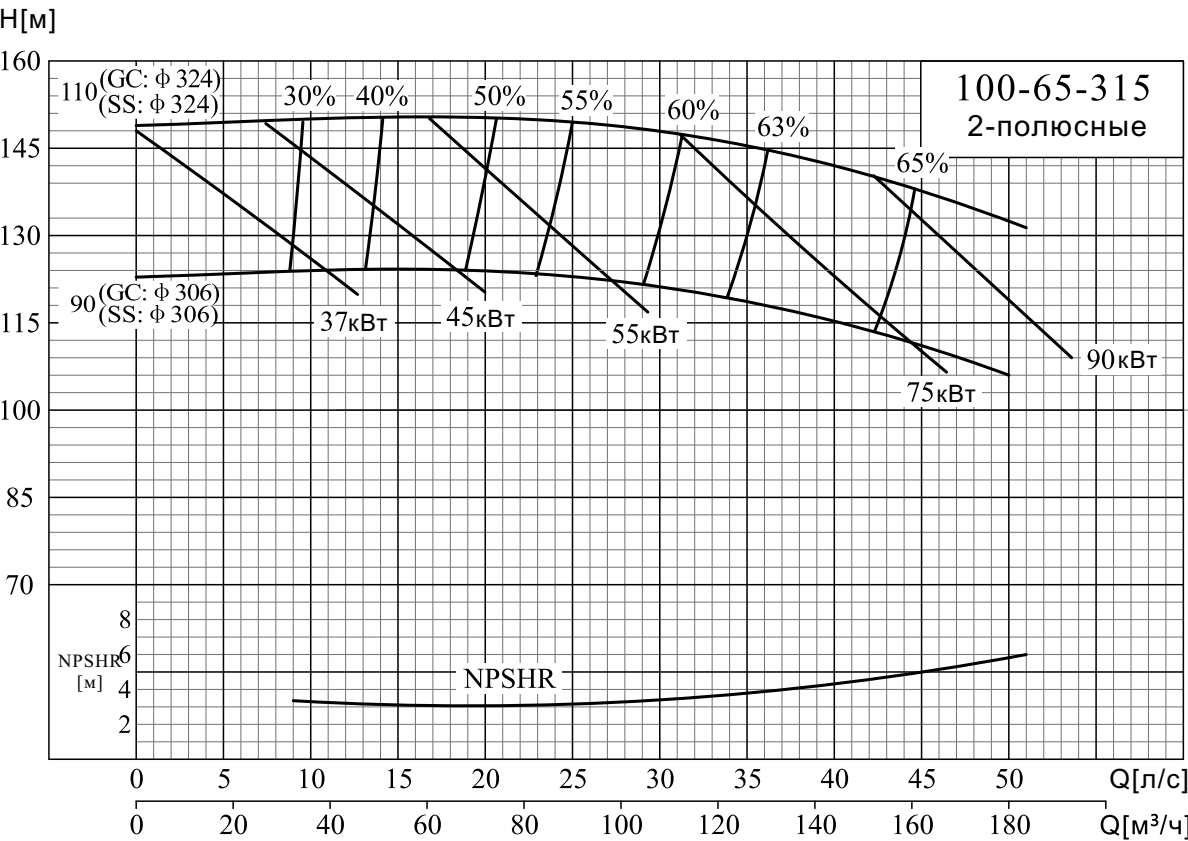
NISO,NIS,NISF100-65-315/100-80-160
