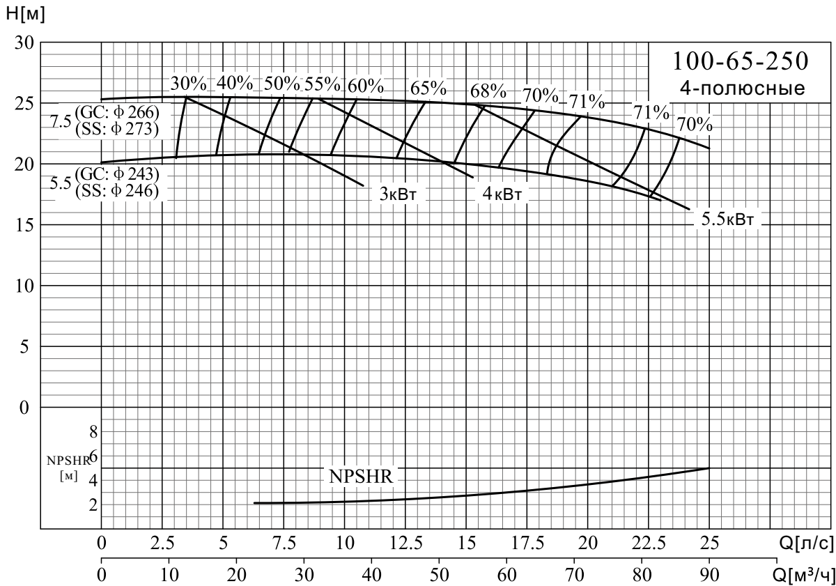
NISO,NIS,NISF 100-65-250/100-65-315
