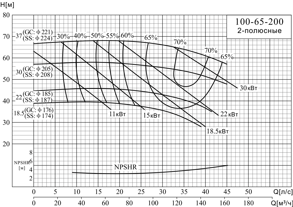
NISO, NIS, NISF 100-65-200/100-65-250
