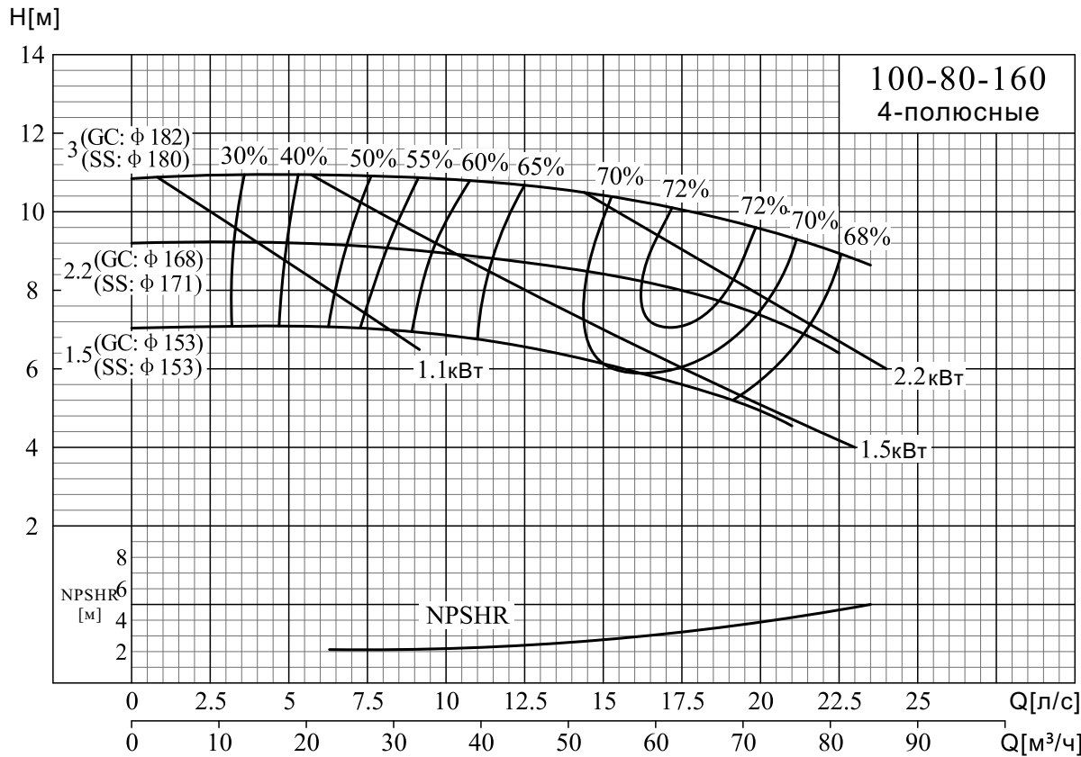
NISO,NIS,NISF 100-80-160/125-100-200
